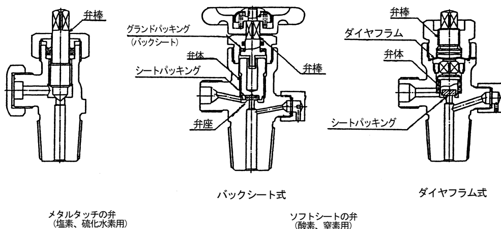
図Ⅱ-6-1 高圧ガス容器弁
